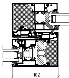
Förhållningspunkt i mittmötet, skala 1:4
